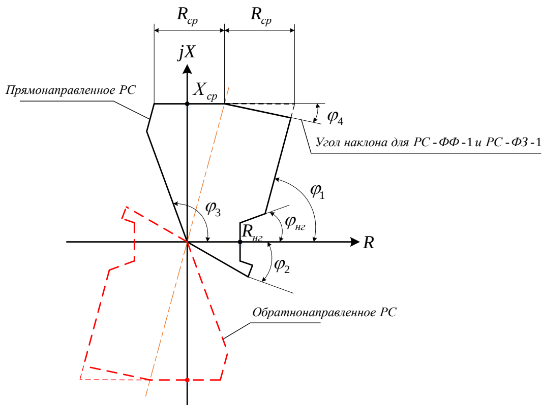
Рисунок 1.4 – Характеристики срабатывания направленного PC
