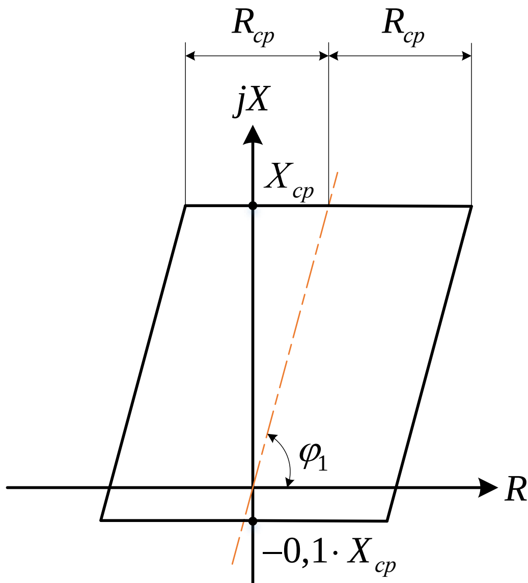
Рисунок 1.5 – Характеристики срабатывания направленного РС
