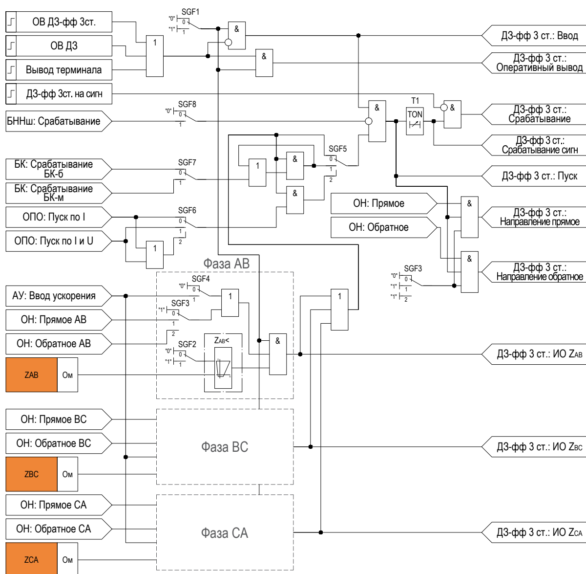
Рисунок 1.8 – Функциональная схема «ДЗ-фф 3 ст.»
