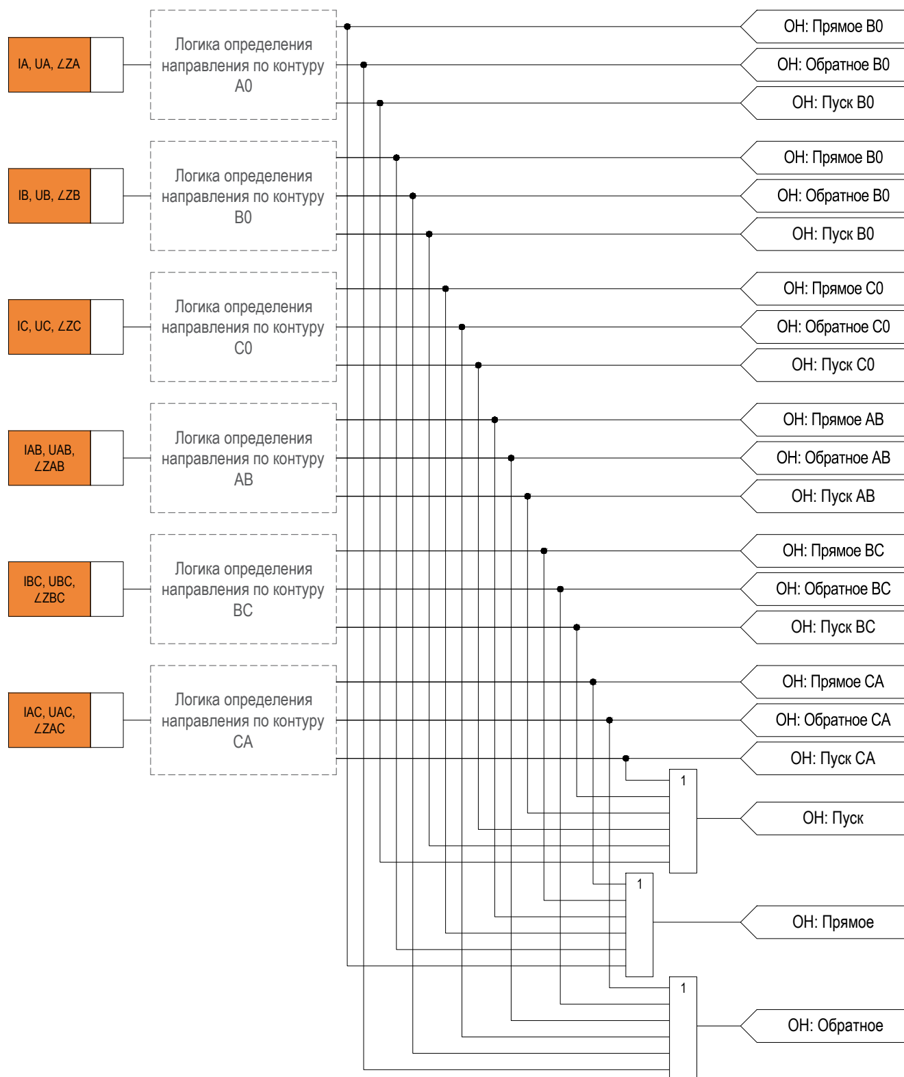
Рисунок 1.13 – Функциональная схема «ОН»
