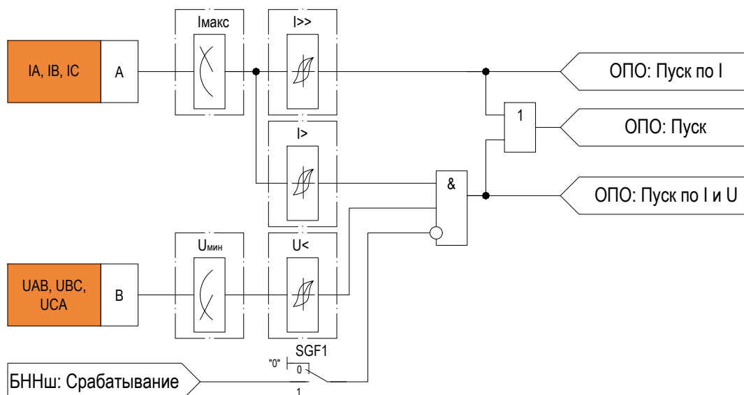
Рисунок 1.14 – Функциональная схема «ОПО ДЗ»
